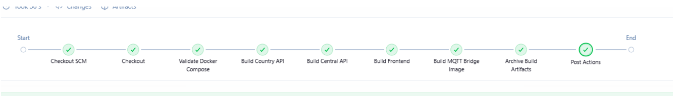
Figure 16 - Job Jenkins FutureKawa-MSPR avec dernier build en succès.
